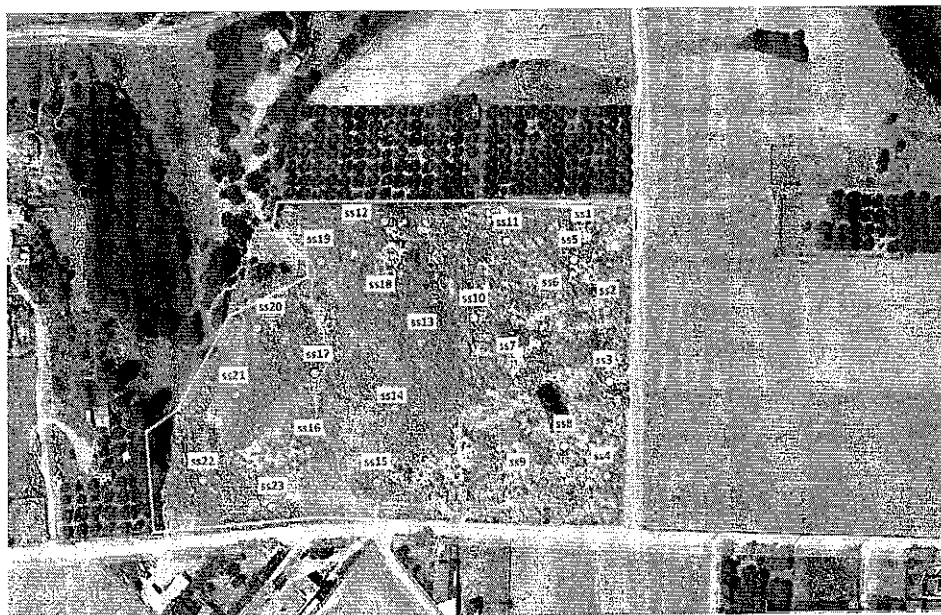
Σχέδιο 1: Θέσεις δειγματοληψίας επιφανειακού εδάφους στην υπό μελέτη περιοχή
