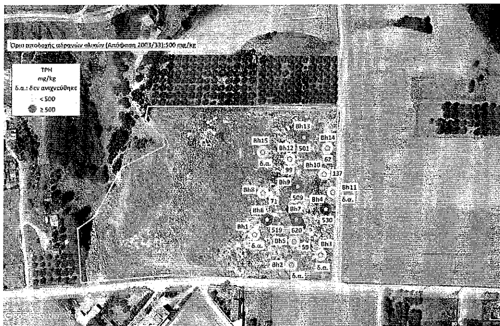
Σχέδιο 5: Συγκεντρώσεις Ολικών Πετρελαϊκών Υδρογονανθράκων (TPH) στα δείγματα εδάφους σε βάθος 0,5 – 1,0 m στην υπό μελέτη περιοχή
