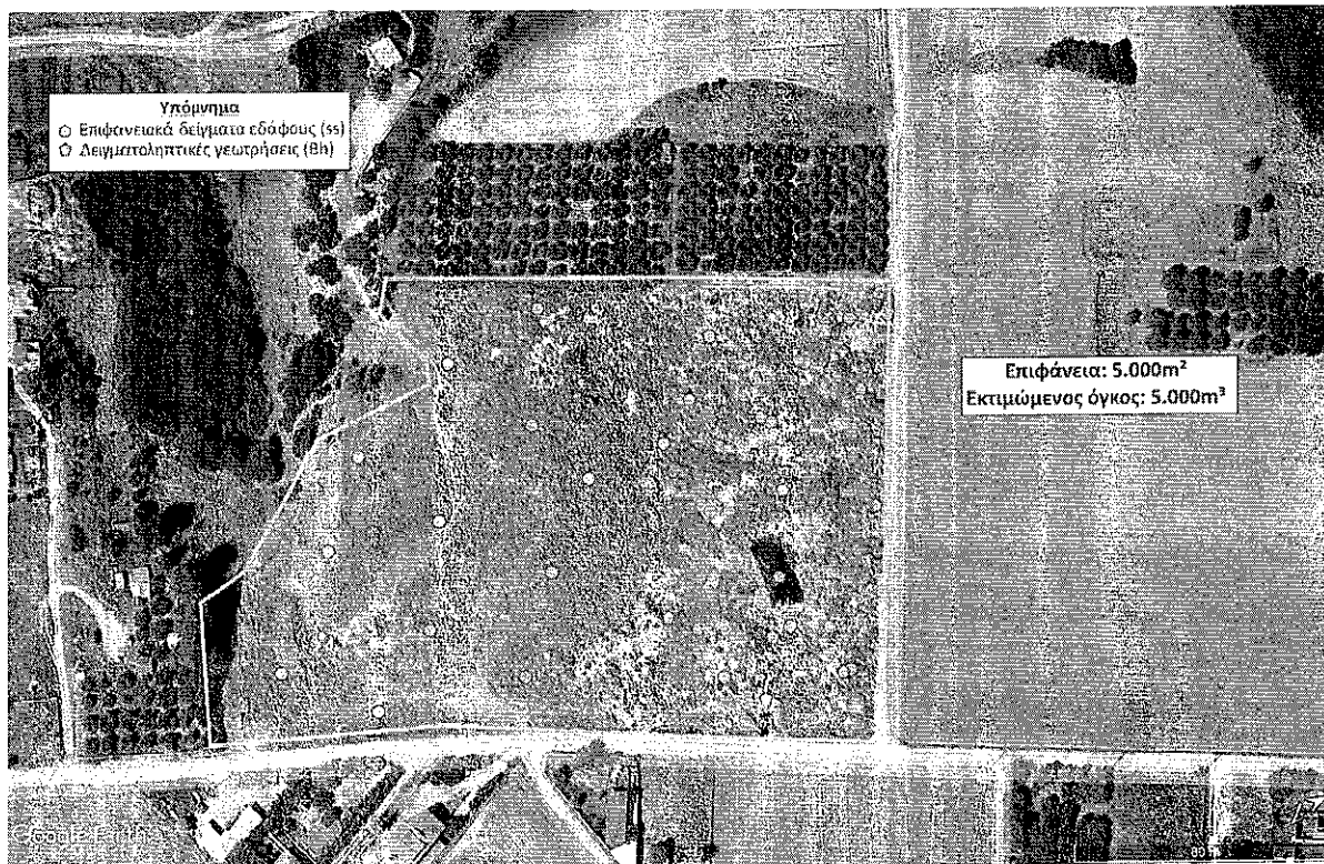
Σχέδιο 7: Εκτιμώμενη έκταση επιβαρυμένου εδάφους από οργανικούς ρύπους
