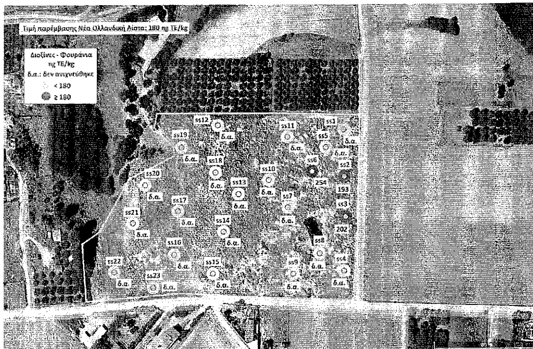
Σχέδιο 3: Συγκεντρώσεις Διοξινών – Φουρανίων στα δείγματα επιφανειακού εδάφους στην υπό μελέτη περιοχή
