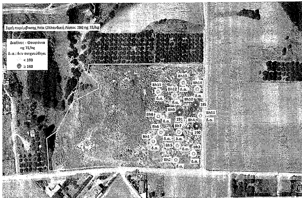
Σχέδιο 6: Συγκεντρώσεις Διοξινών – Φουρανίων στα δείγματα εδάφους σε βάθος 0,5 – 1,0 m στην υπό μελέτη περιοχή
