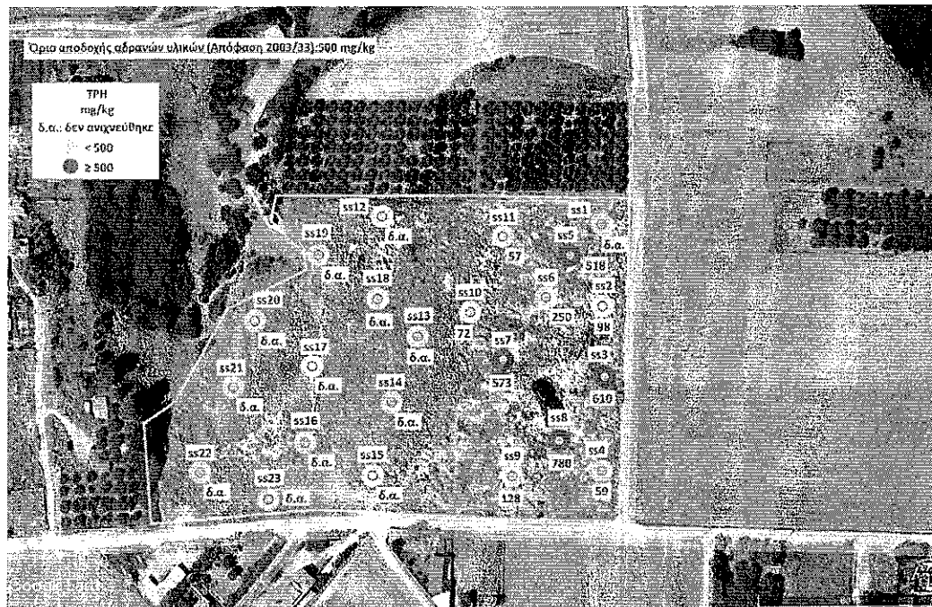
Σχέδιο 2: Συγκεντρώσεις Ολικών Πετρελαϊκών Υδρογονανθράκων (TPH) στα δείγματα επιφανειακού εδάφους στην υπό αποκατάσταση περιοχή
