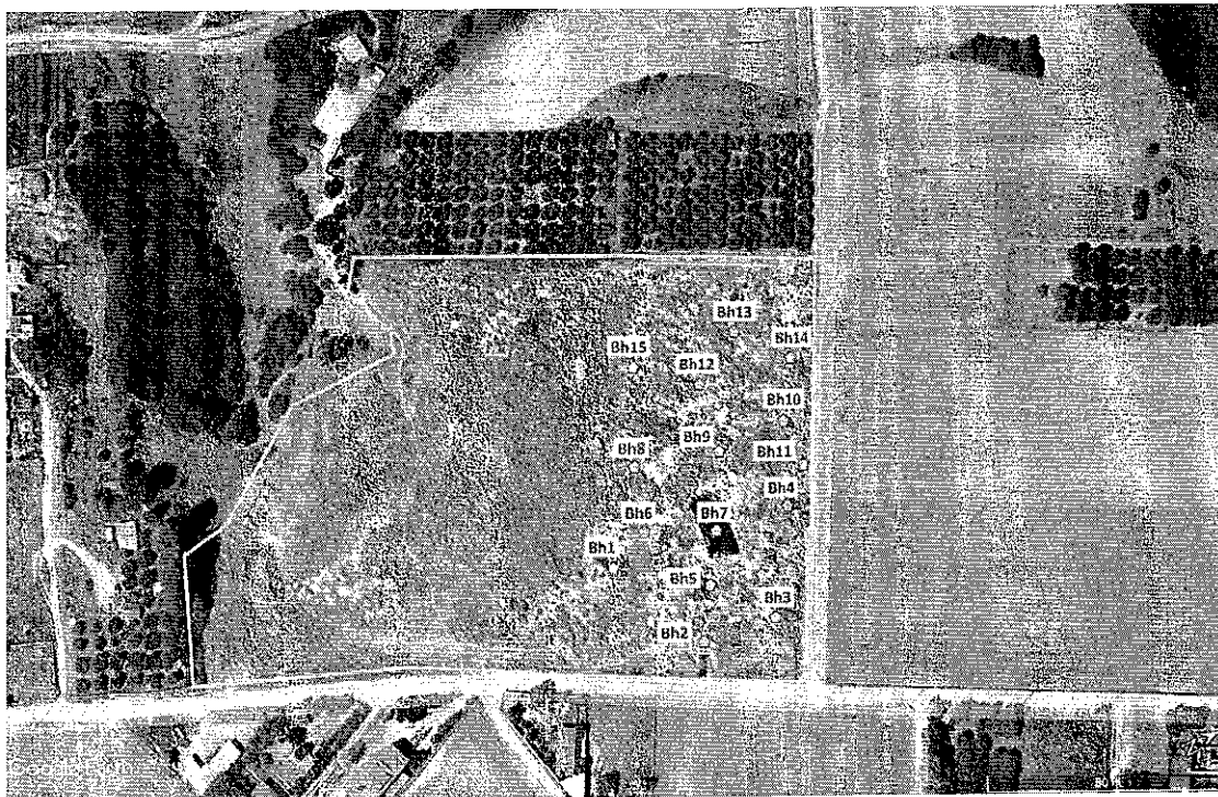
Σχέδιο 4: Θέσεις δειγματοληπτικών γεωτρήσεων στην υπό μελέτη περιοχή
