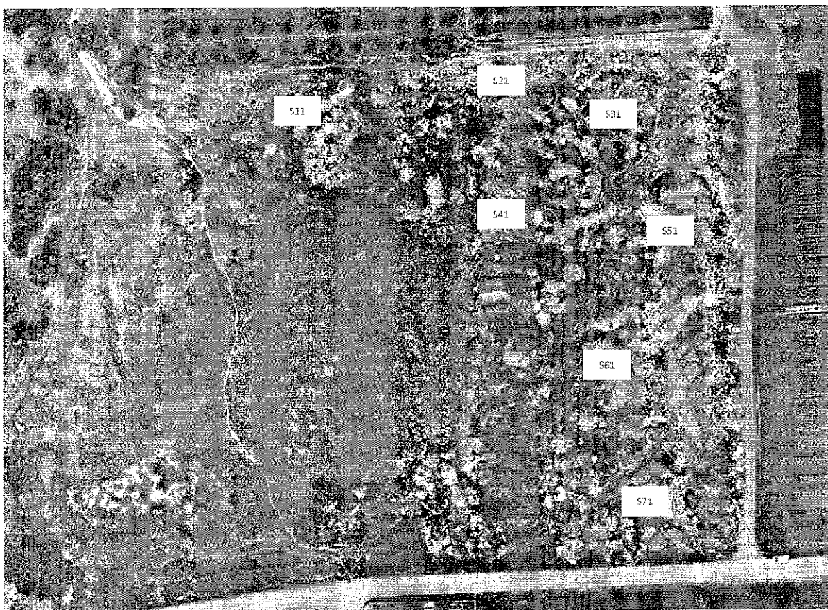
Εικόνα 8: Θέσεις δειγματοληψίας επιφανειακών χωμάτων
